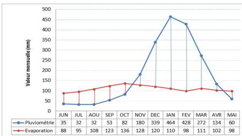
FIGURE 8. COURBES « PRÉCIPITATION - ÉVAPORATION » A NOSY BE (MOYENNES MENSUELLES)
